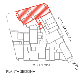
PLANTA SEGONA
